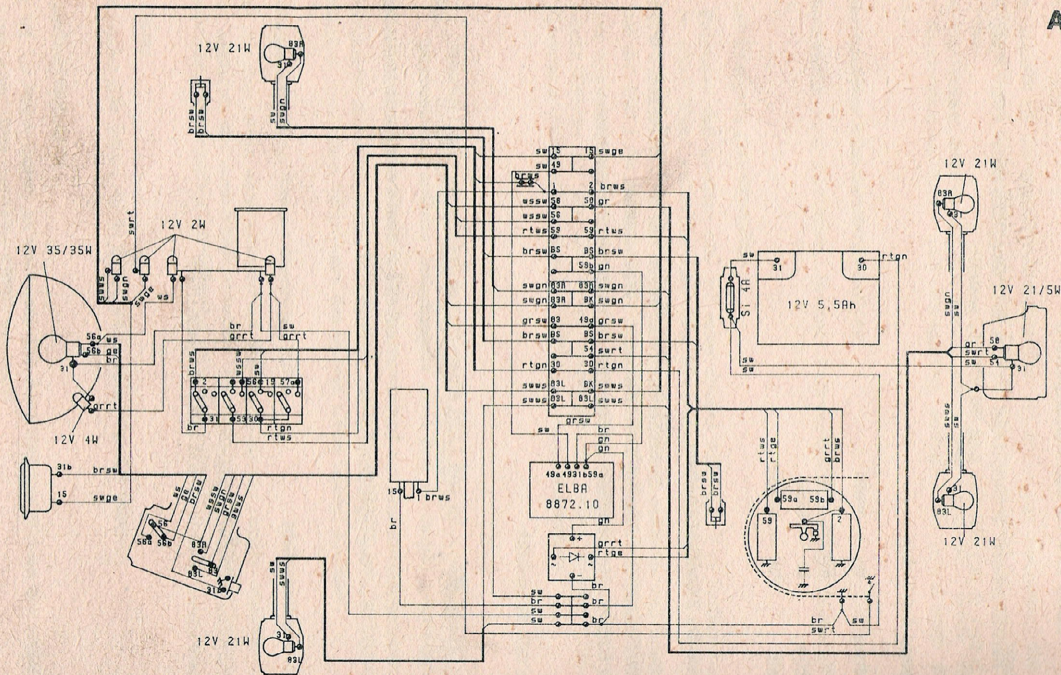
Bild 214. Schaltplan für SR 50/1 B
