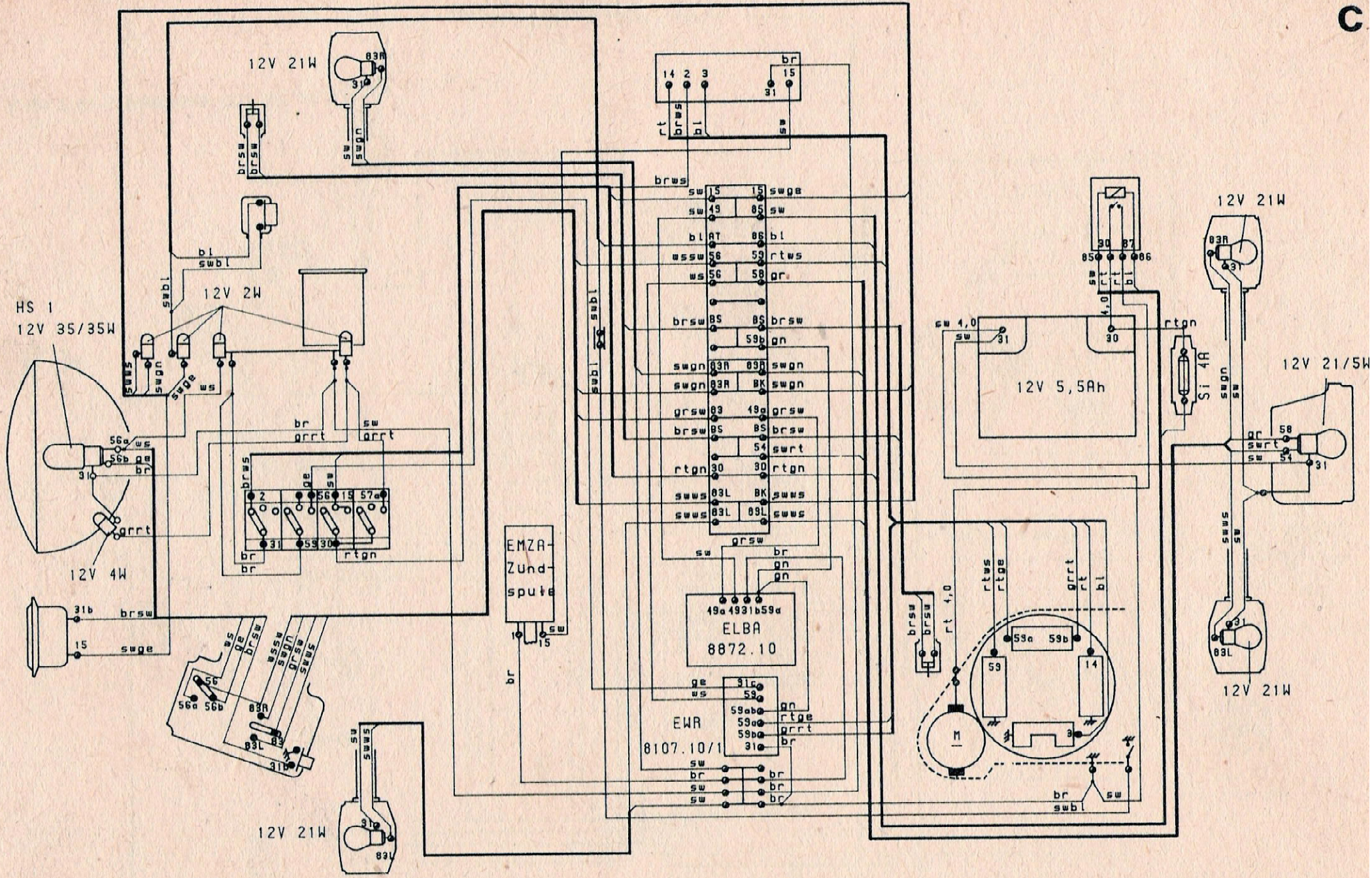
Bild 216. Schaltplan für SR 50/1 CE und SR 80/1 CE
